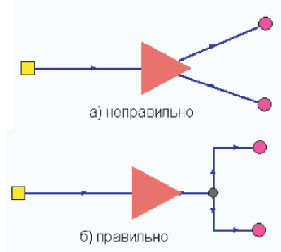
Рисунок 7.9 - Отображение ЦТП
